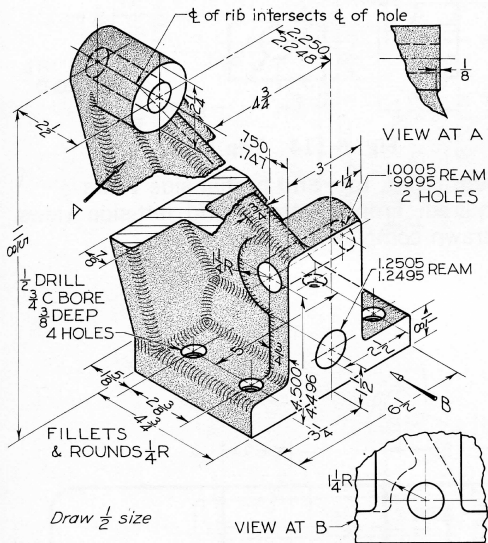
Fig. 6-109 Ejector Base (Layout C-4).*
