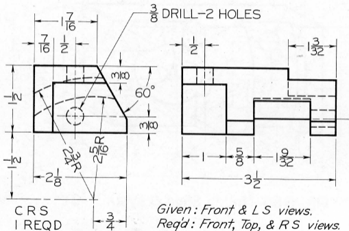
Fig. 6-73 Shifter Block (Layout A-3).*
