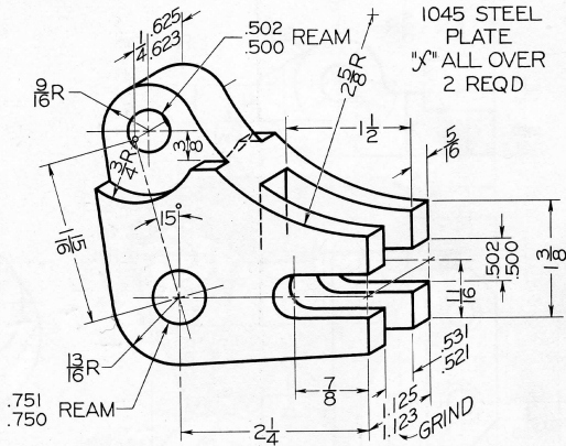
Fig. 6-66 Toggle Lever (Layout A-3).*
