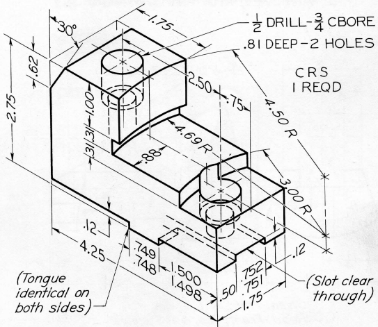
Fig. 6-70 Chuck Jaw (Layout A-3).*
