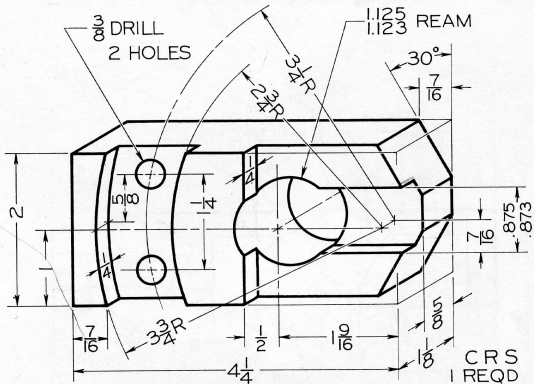
Fig. 6-68 Index Slide (Layout A-3).*
