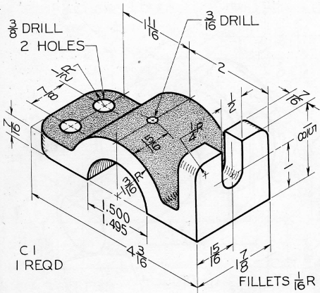
Fig. 6-69 Frame Guide (Layout A-3).*
