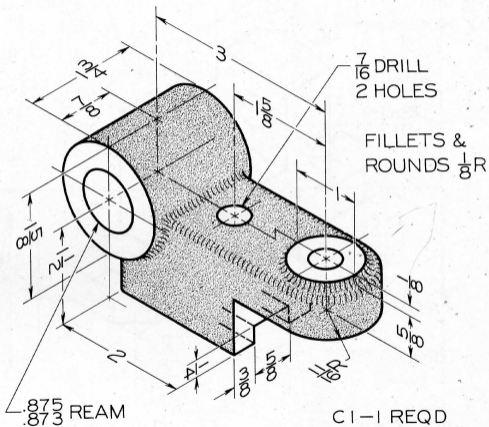
Fig. 6-62 Index Arm (Layout A-3).*
