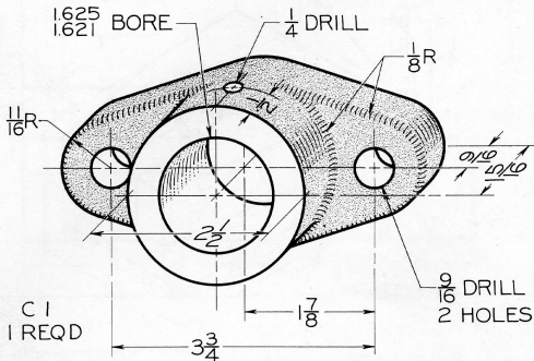
Fig. 6-59 Bearing (Layout A-3).*
