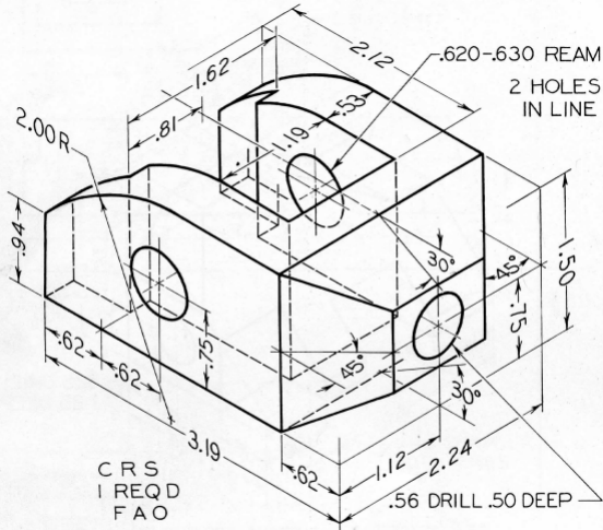
Fig. 6-61 Cam (Layout A-3).*
