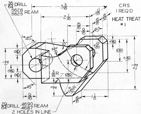
Fig. 6-63 Roller Lever (Layout A-3).*
